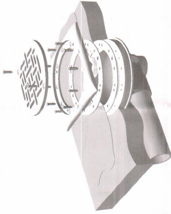
Assemblage sur piscine béton et liner Concrete pool with liner assembly Montaje piscina hormigon con liner
